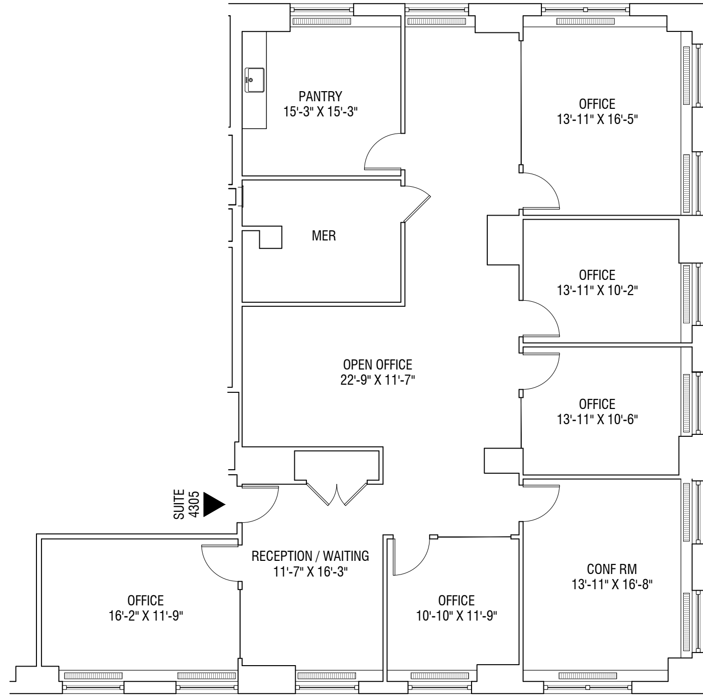
1 SUITE 4305 EXISTING SCALE: 1/8" = 1'-0"
