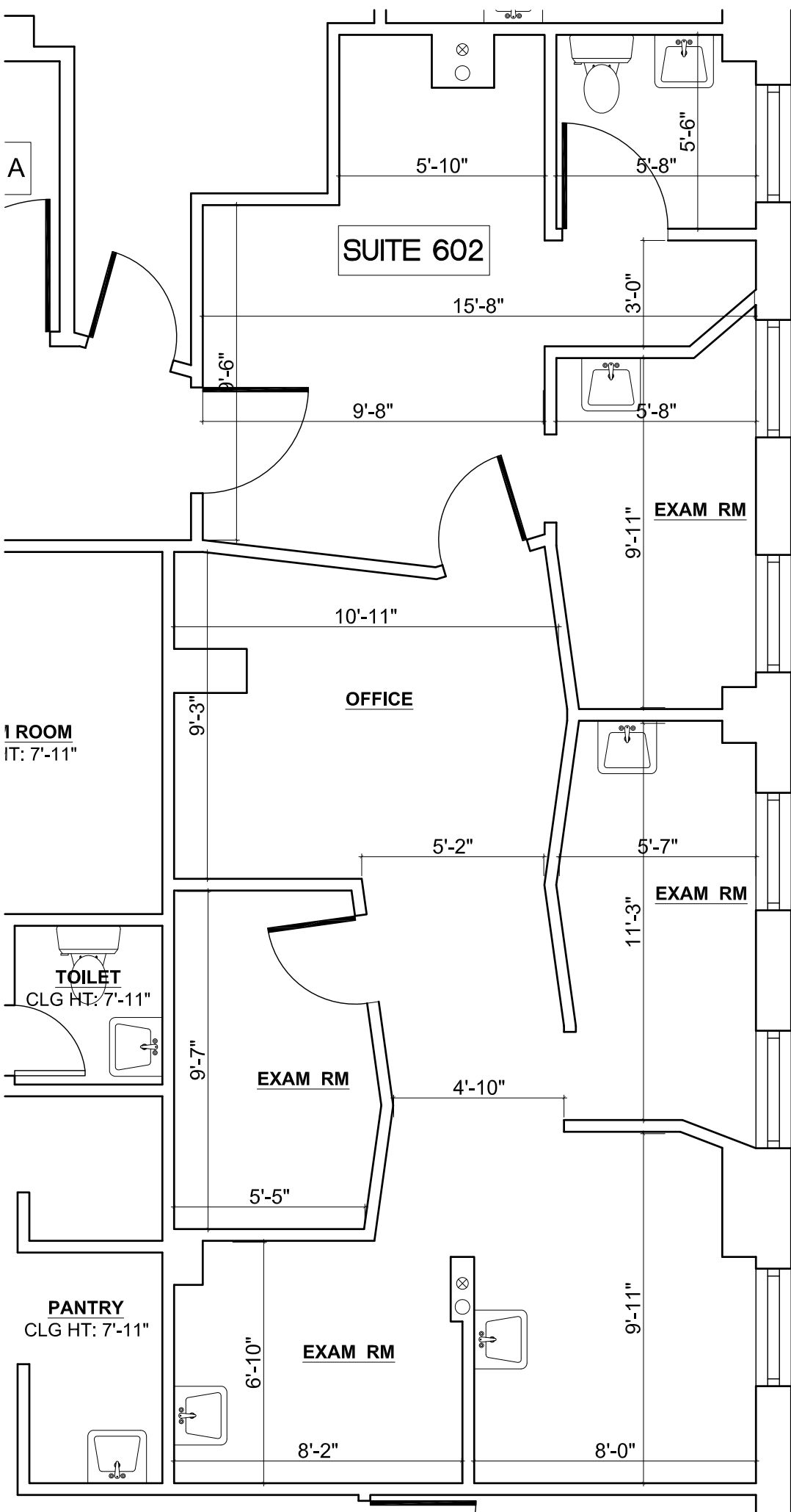
SUITE 602 SCALE: 1/4"=1'-0"
